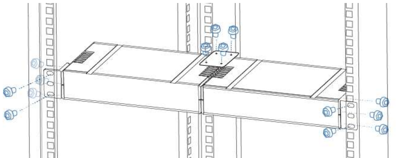
图1 两台设备并列安装示意图（使用短挂耳）
